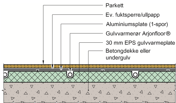
Fig. 4 Arjonfloor Golvvarmerør i spor i Easy polystyrenplater
