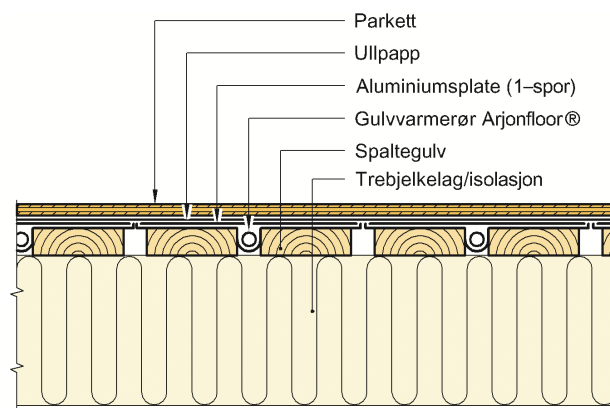
Fig. 6 Arjonfloor Golvvarmerør lagt i spor i varmfeddelingsplate i spaltegolv
