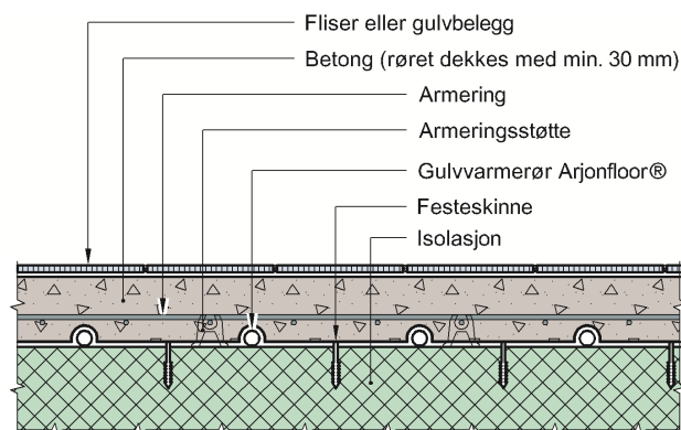
Fig. 2 Arjonfloor Golvvarmerør festet med festeskinne og innstøpt i betong eller avrettingsmasse. Overdekning over varmerørene skal være minimum 30 mm.
