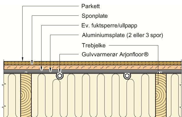
Fig. 5 Arjonfloor Golvvarmerør lagt i spor i varmfeddelingsplate på trebjelkelag.
