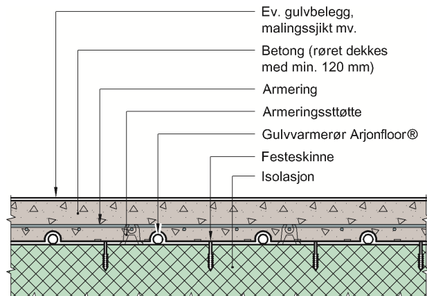
Fig. 3 Arjonfloor Golvvarmerør festet med festeskinner i industrigolv
