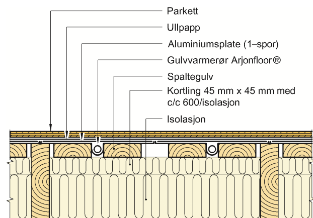
Fig. 7 Arjonfloor Golvvarmerør lagt i spor i varmfeddelingsplate i et spaltegolv som er senket i forhold til overkant bjelkelag
