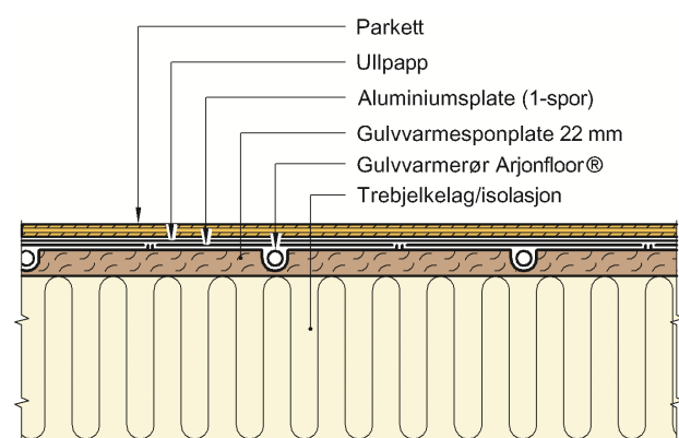
Fig. 8 Arjonfloor Golvvarmerør lagt i spor i sponplate over trebjelkelag.
