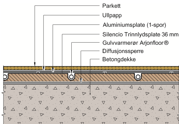
Fig. 9 Arjonfloor Gulvvarmerør i Silencio trinnlydsplate på bærende underlag av betong
