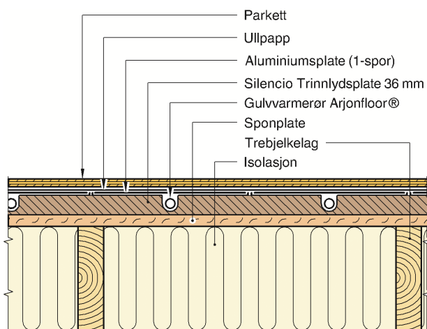
Fig. 10 Arjonfloor Gulvvarmerør i Silencio trinnlydsplate på bærende underlag av sponplater
